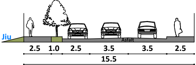
Str. 1 Decembrie 1918 profil CC'
