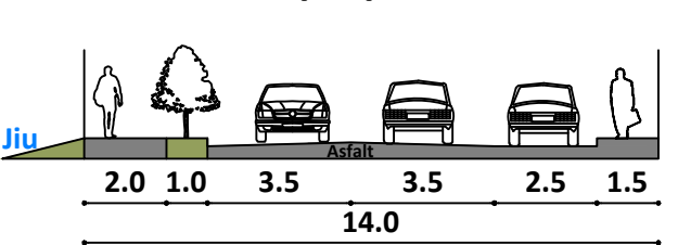
Str. 1 Decembrie 1918 profil AA
