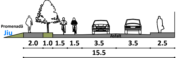
Str. 1 Decembrie 1918 profil BB'
